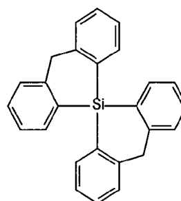
9,9-spirobissilaanthracene
