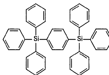
p\text{-(SiPh}_3)_2\text{Ph}
